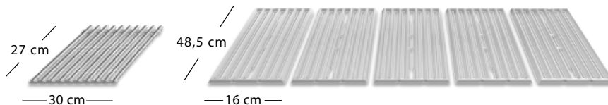
Massive Edelstahlgrüsse
